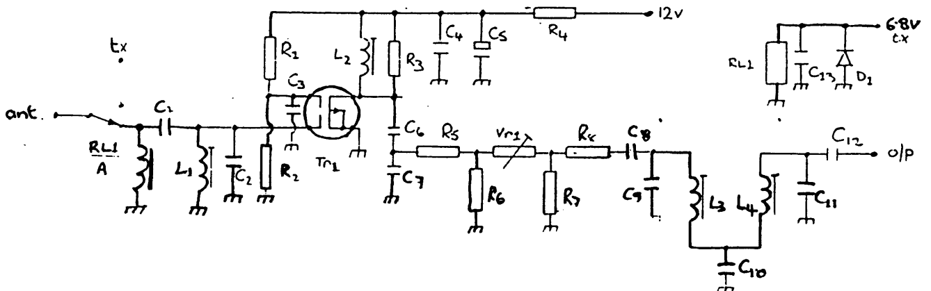
Circuit schematic SLNA 145sb
